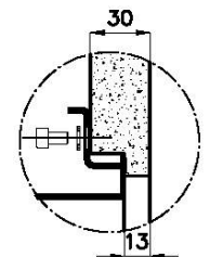
A-A: Dettaglio installazione positive reveal e sistema di fissaggio Installation detail with positive reveal and fixing system
